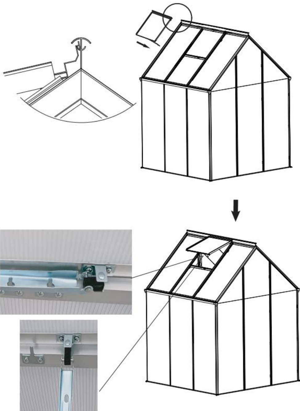
Монтаж на плъзгаща се врата
